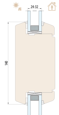
NATURO 68 SYSTEEM structurele roede 140 mm
