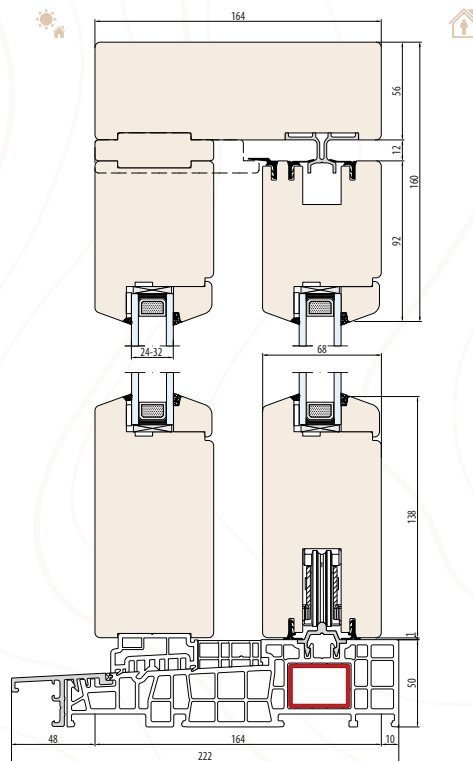
NATURO 68 HST SYSTEEM (algemene afmetingen) - drempel 50 mm - schema "A"
