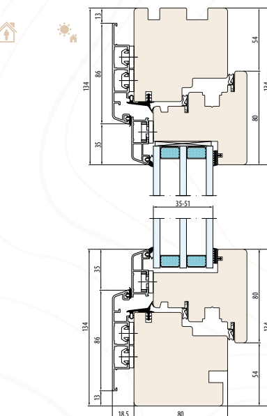
NATURO 80 ALU SYSTEEM GEMINI CLASSIC interne afsnijding onder het raamkozijn
