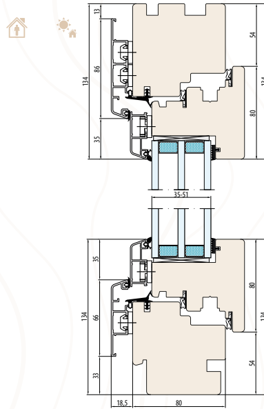
NATURO 80 ALU SYSTEEM GEMINI CLASSIC interne en externe afsnijding onder het raamkozijn
