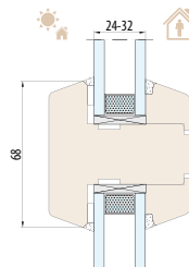
NATURO 68 SYSTEEM structurele roede 68 mm
